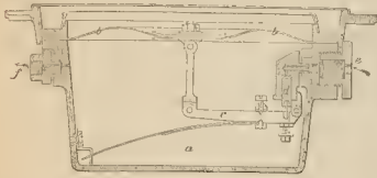
Fig. 1. Regulador para el alumbrado por gas comprimido
